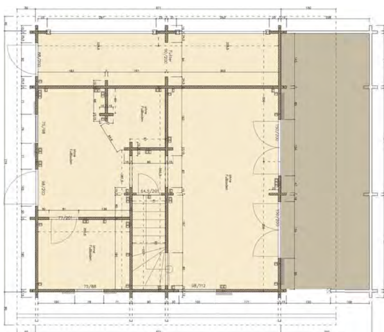
GRUNDRISS EG
